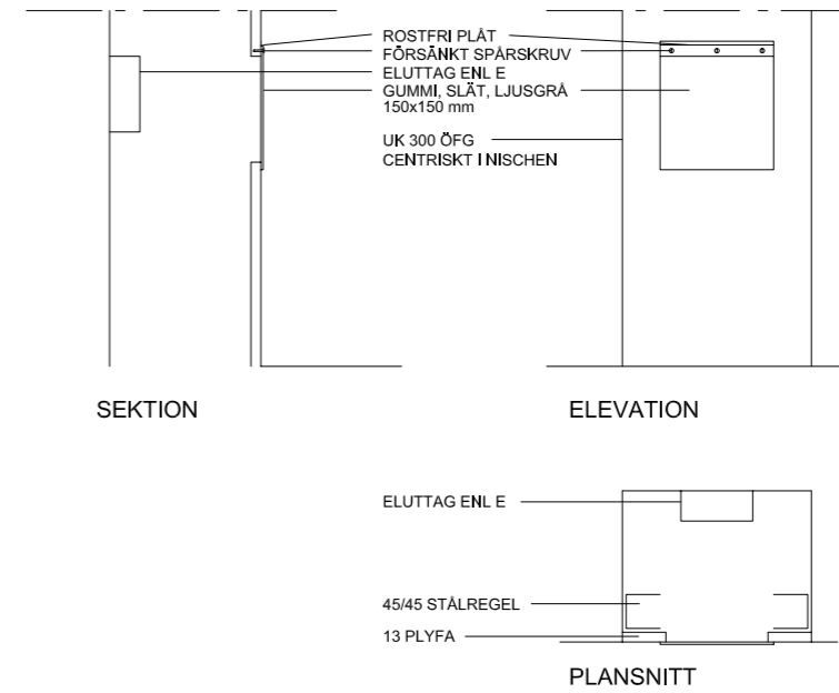
DETALJ "EU" GÖMDA ELUTTAG I BEF NISCHER
