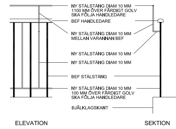
DETALJ "BA" KOMPLETTERING BARNSÄKERHET - RÄCKEN
