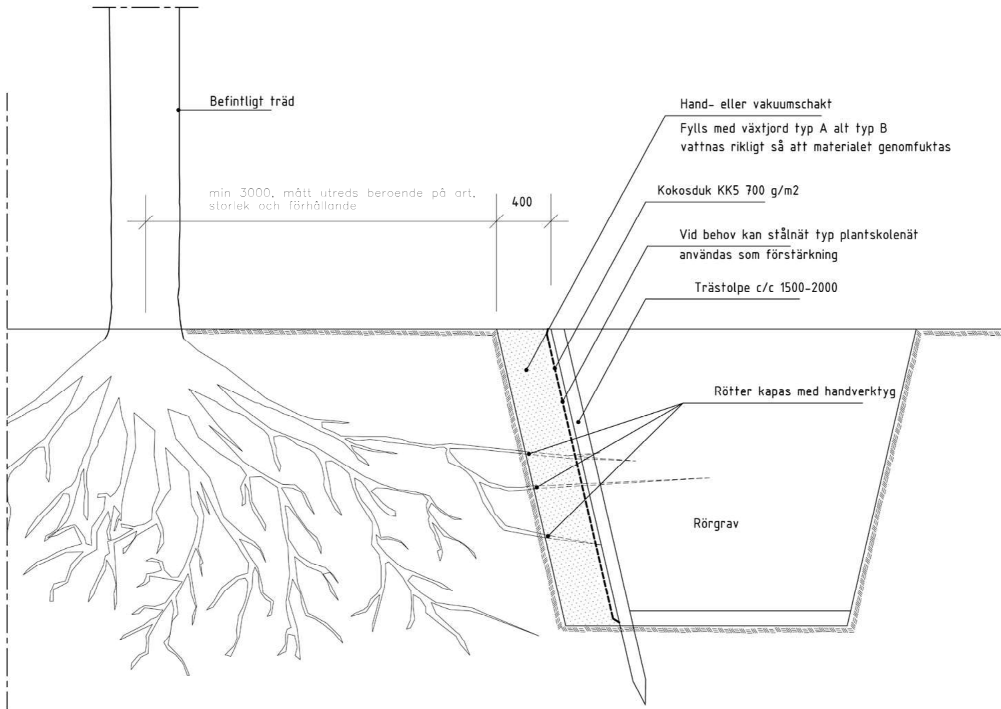
SEKTION ROTDRAPERI SKALA 1:20 (A2), 1:40 (A4)
